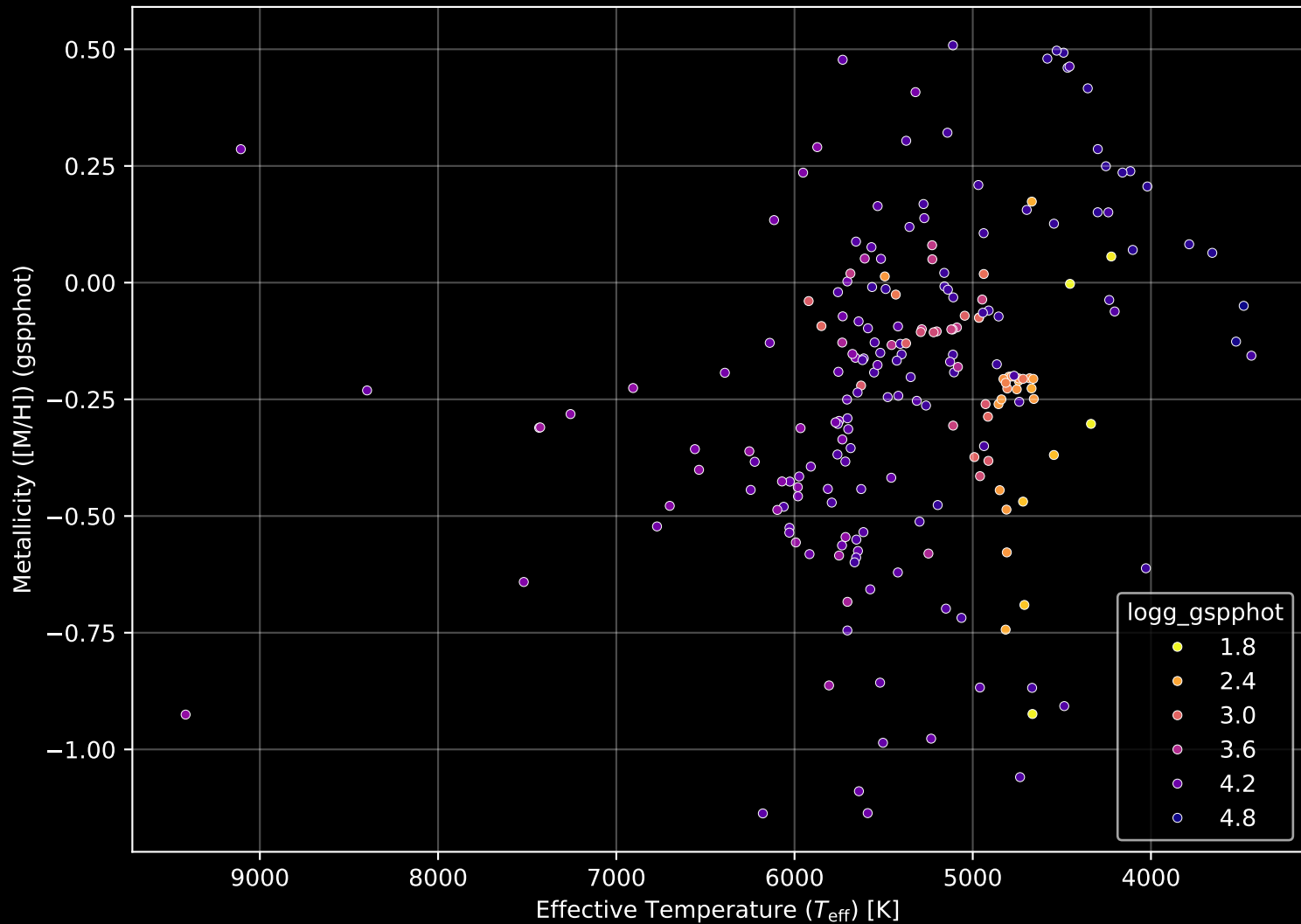
APOGEE DR17 Field: [135-30] Stellar Population Parameters (n= 211)
